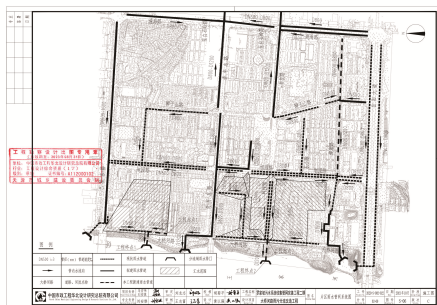
大桥河路管网总平面布置图
