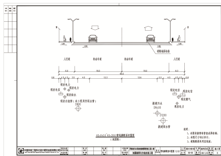
旭园路管线横断面示意图
