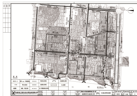
旭园路管网总平面布置图
