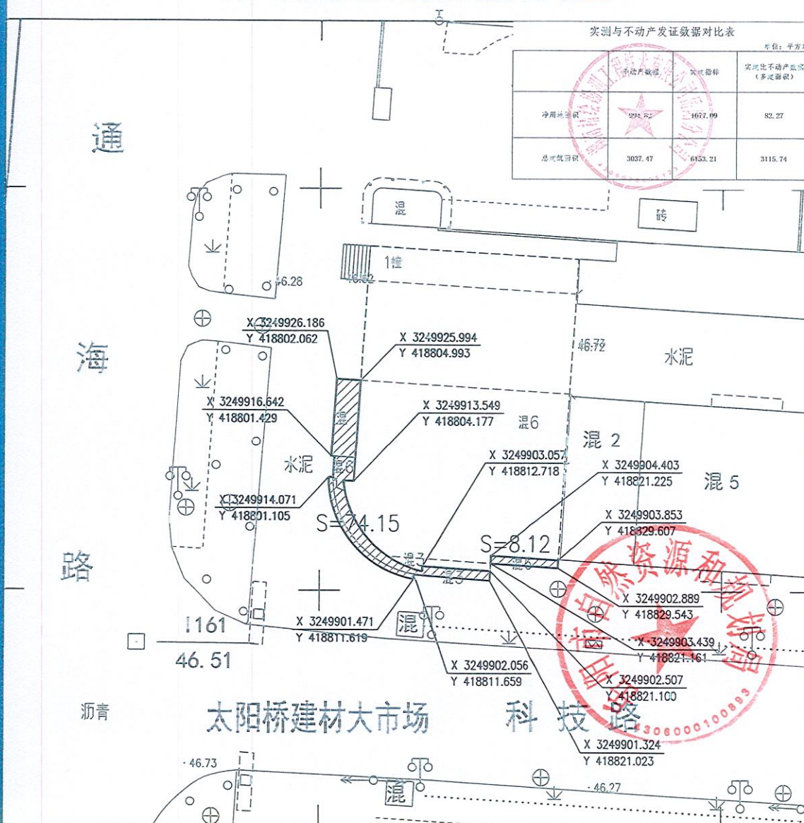
太阳桥建材大市场1栋西152、153、252、253、352、353号3层 商业楼违法扩建项目现状审批图
